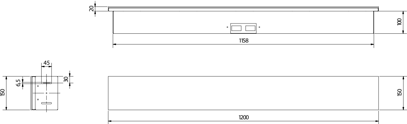
» INFOBAR technical drawing - Pic. 2 «
